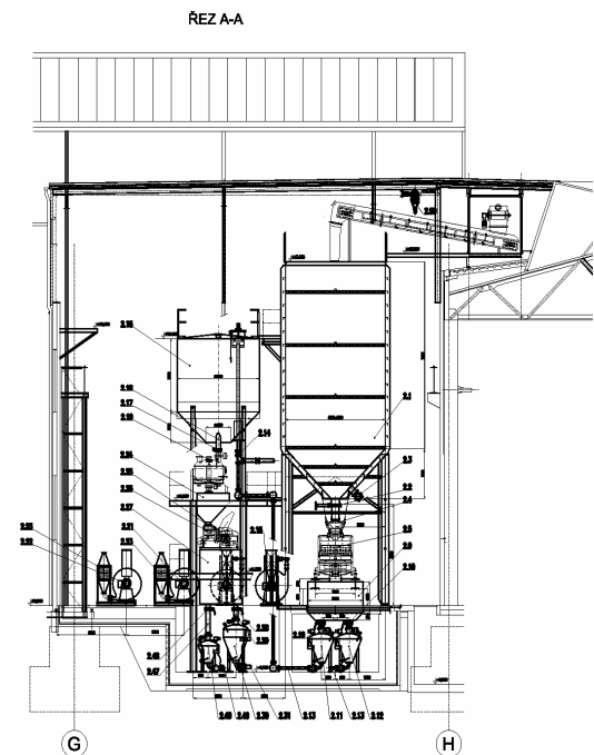
Drcení a chlazení vratu, I.separace chromitu
