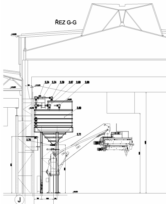
Zásobník s míšičem Wöhr
