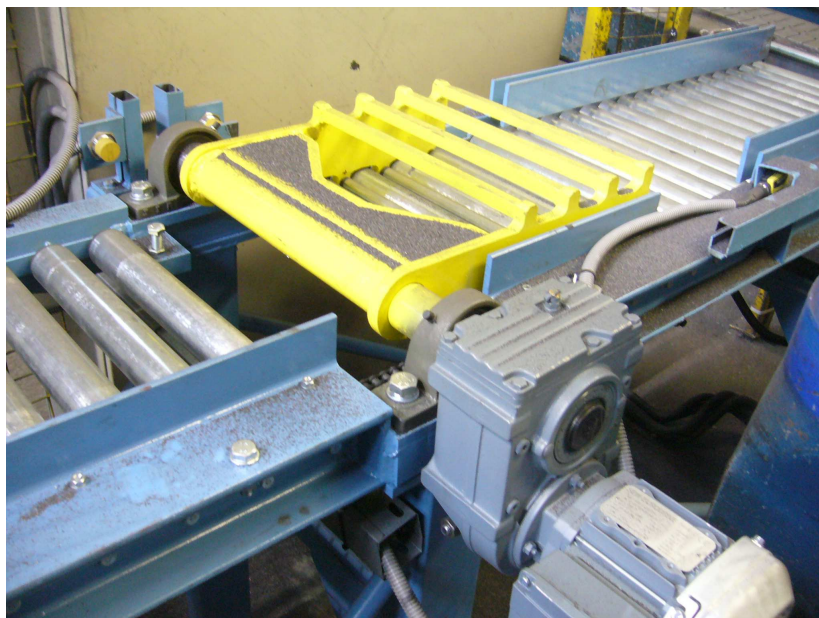
Pohled na obraceč kotoučů
